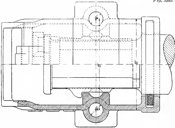
Fig. 5383. Longitudinal Section.
